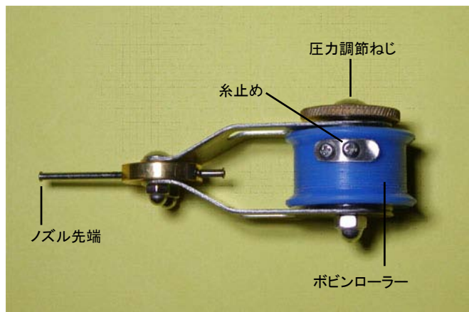
パッカー各部分名称
